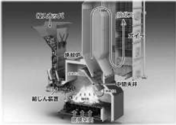
▲ストーカ式焼却炉の構造
